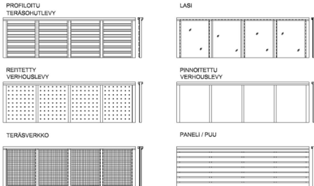
Kuva 8 Esimerkkejä kevyistä kaideratkaisuista.
