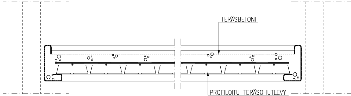
Kuva 7 Liittolaattarakenne.
