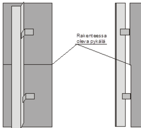
Kuva 6 Säätökiinnikkeiden periaate.
