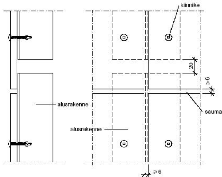
Kuva 7 Esimerkki levyn kiinnityksestä rankarakenteen jatkoskohdassa.
