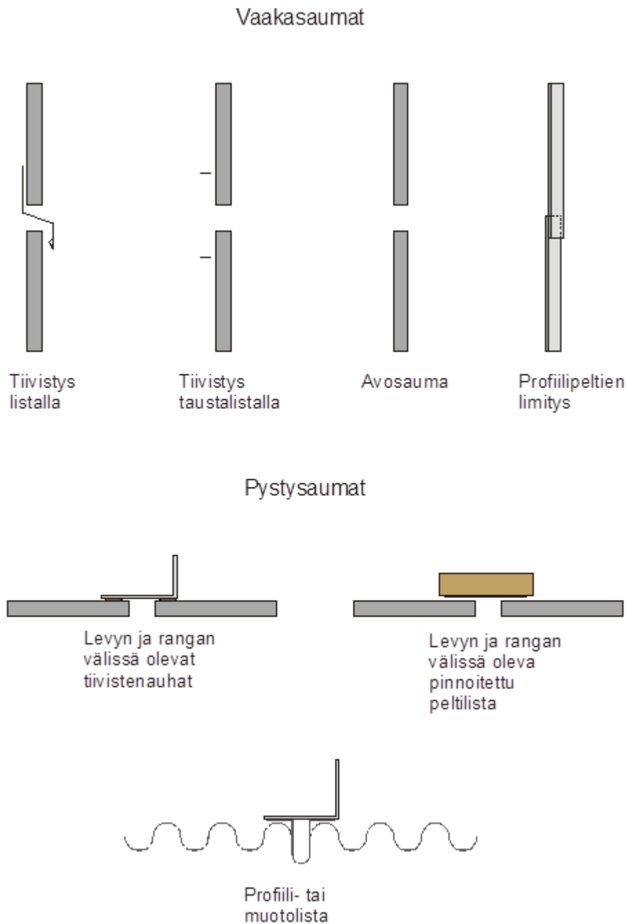
Kuva 11 Periaatteellisia levyjulkisivun saumaratkaisuja.
