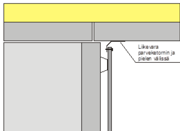
Kuva 13 Periaatekuva parvekepielen verhouksen liittymästä ulkoseinään.
