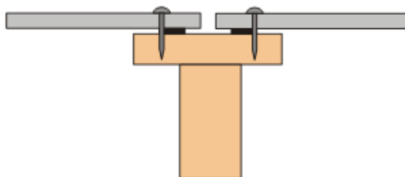
Kuva 4 Tiivisteet puun ja julkisivulevyn liitoskohdassa.
