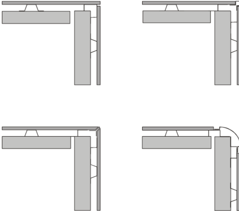
Kuva 12 Erilaisia ulkonurkkaliitoksia.
